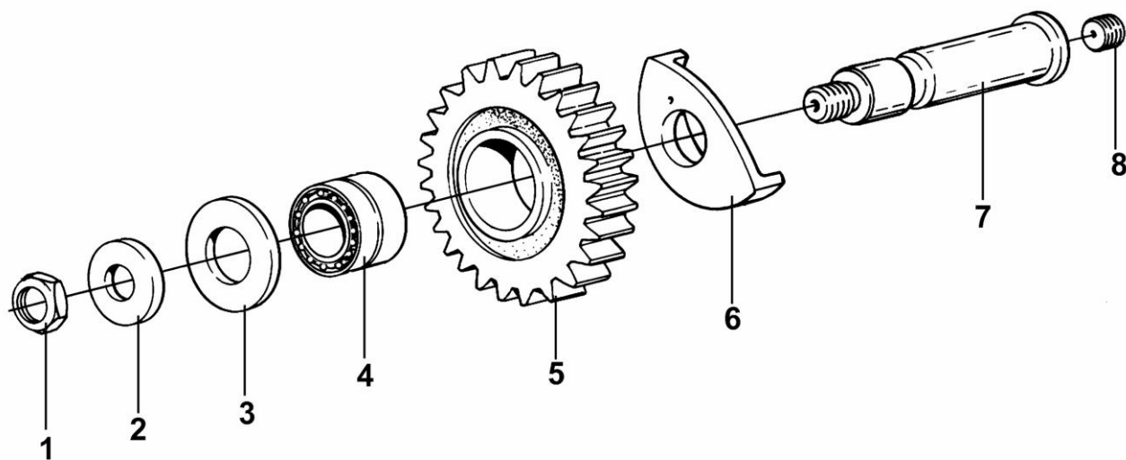
倒挡总成爆炸图
