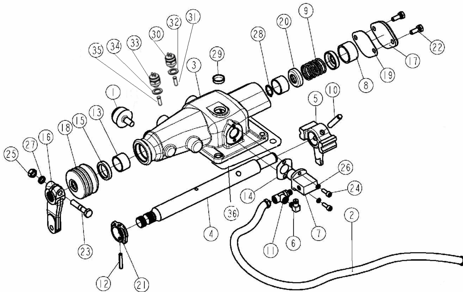
换挡操纵机构爆炸图
