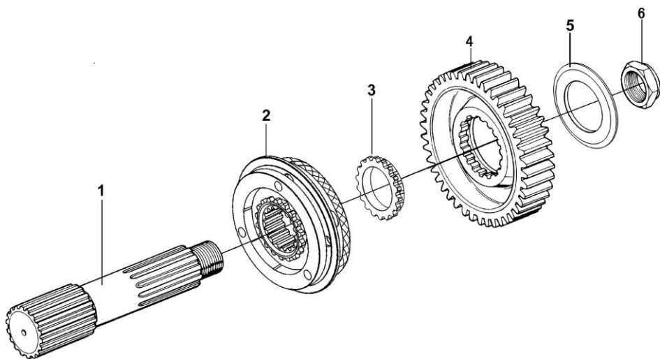
副箱主轴总成爆炸图
