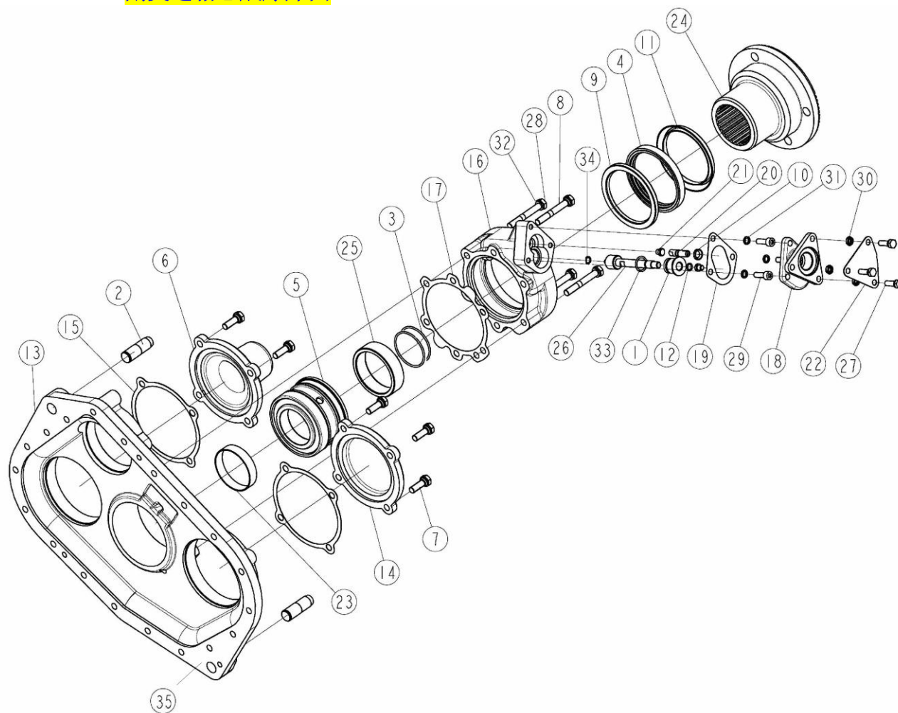
副变速箱总成爆炸图
