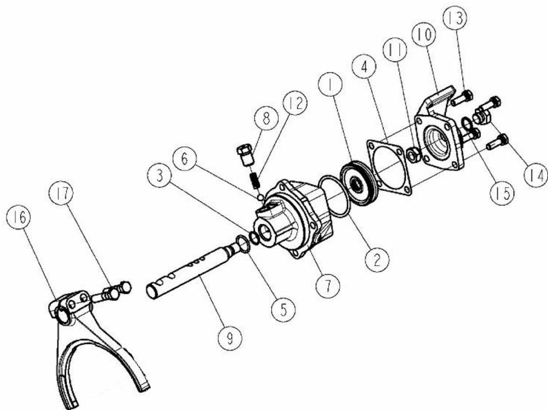
副箱换挡汽缸总成爆炸图
